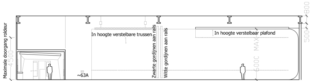
Langsdoorsnede
